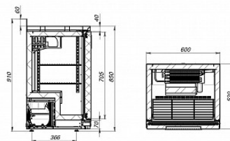
Ствол барный TM101/Гельховая дверь и столешница с бортом!
